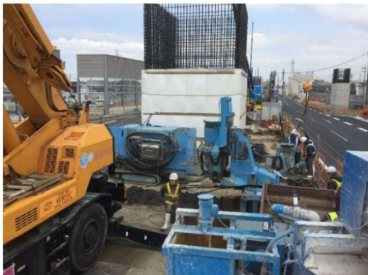
国土省愛知国道事務所 環西蟹田南高架橋下部工事
