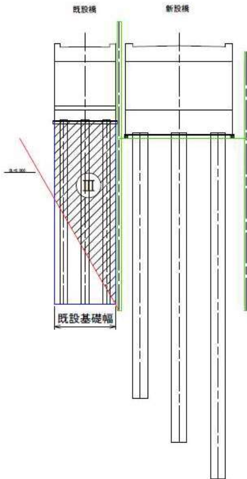
土留め壁の引抜きによる影響範囲
