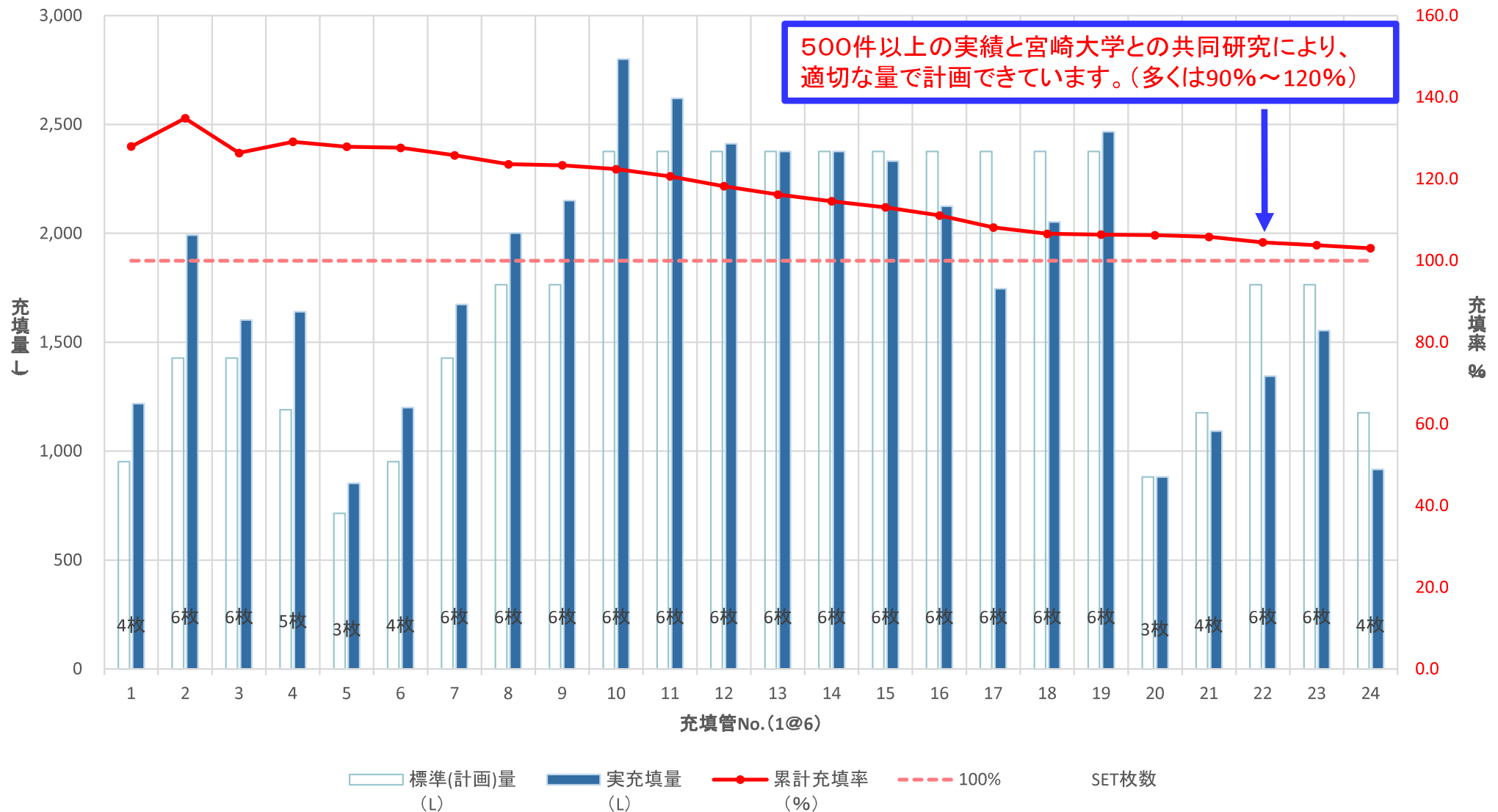
●●村充填量管理グラフ(施工事例)
