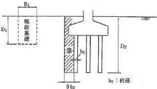
図2-1 場所打ち杭基礎の場合の影響範囲
